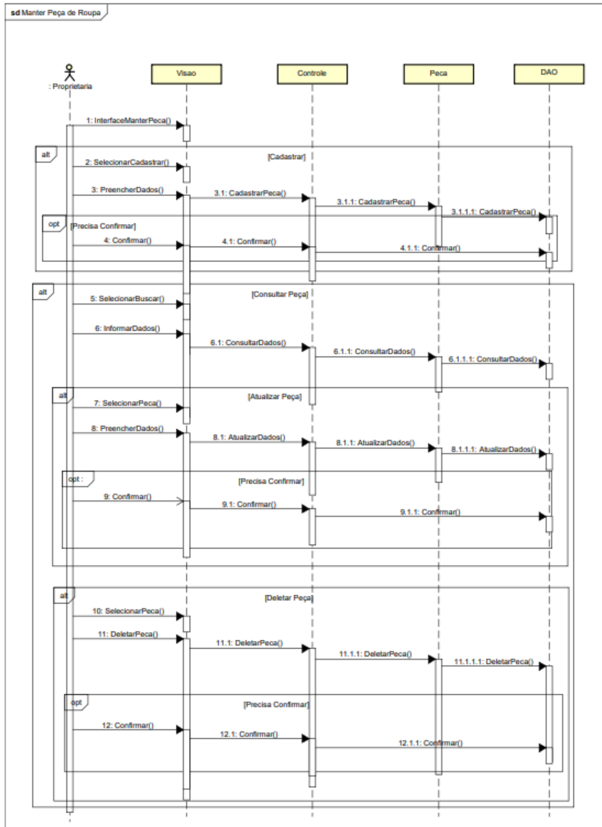
Figura 5 – Diagrama de sequência de peça de roupa
