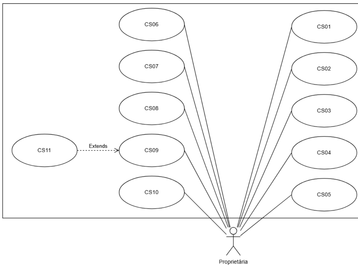
Figura 1 – Casos de Uso do sistema “Minha Lojinha”
