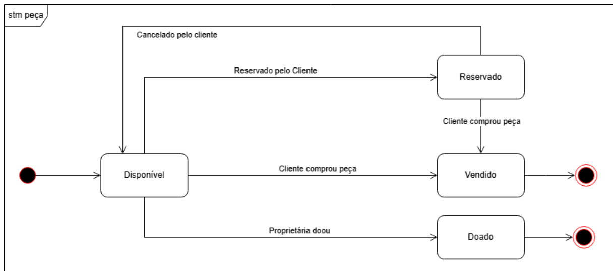
Figura 3 – Diagrama de estados de peça
