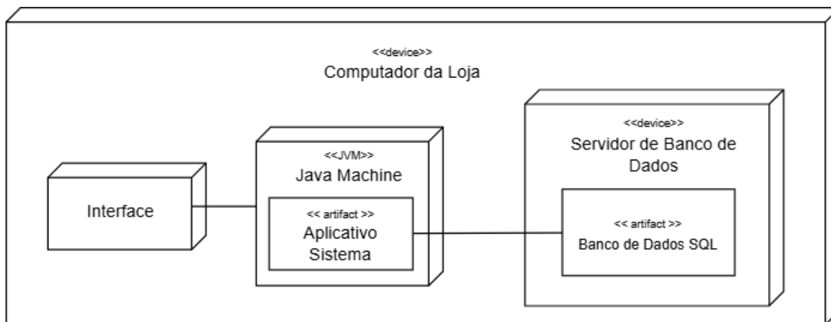
Figura 8 – Diagrama de Implantação do sistema “Minha Lojinha”
