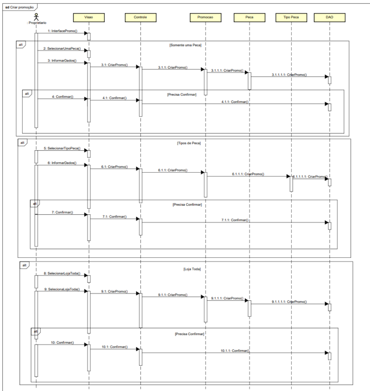
Figura 7 – Diagrama de sequência da criação de promoções da loja
