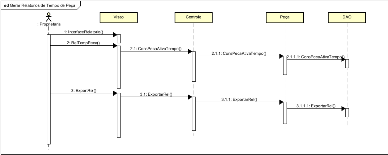
Figura 6 – Diagrama de sequência da geração de relatórios de tempo de peça
