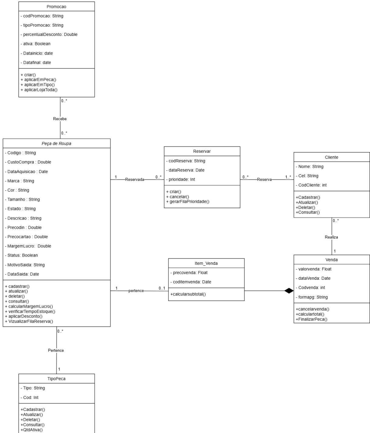
Figura 2 – Diagrama de Classes do sistema “Minha Lojinha”
